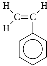
styrene
